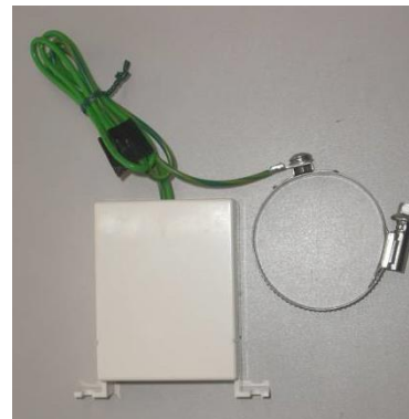
ITB (Ion Tuning Box) (コンデンサーに同梱されていません) (交換の目安は5年です)
